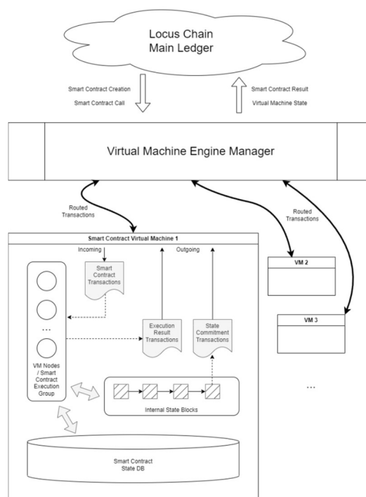
Figure 9: 로커스체인 VME 구조
